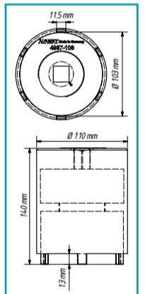
Drážkovaná matice
