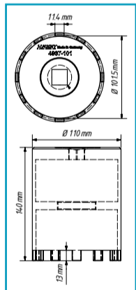
Drážkovaná matice
