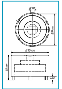
Drážkovaná matice
